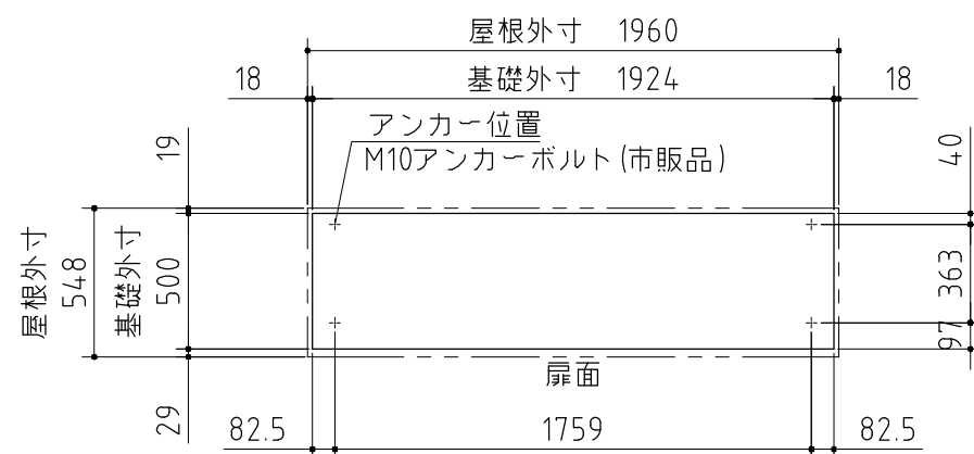
ベタ基礎図
